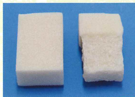
断熱材への影響を実験。 左がペネザープに浸漬した もの、右の変形している方は 『油溶剤』という油ベースの 薬剤に浸漬させたものです。
